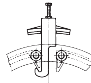
cable clamp LK
